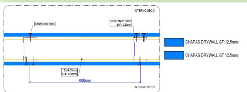
PAR TIPO 1 - Esp. 9,5cm - Planta
