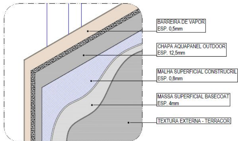
Sistema AQUAPANEL - espessura das camadas
