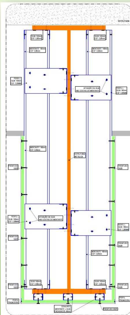
DETALHE 28 - Aquapanel - Corte Esc. 1:5
