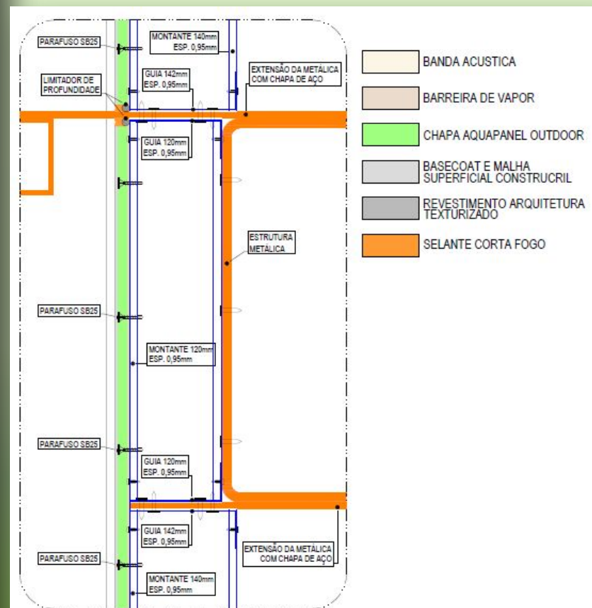
DETALHE 27 - Aquapanel x metálica - Corte Esc. 1:5
