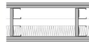
Figura 27 – Colocação da lâ de rocha em paredes com dupla estrutura ligada – fonte: Manual de projeto e sistemas de drywall – Fonte: Associação Drywall
