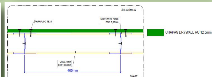
PAR TIPO 6 - Esp. 8,25cm - Planta
