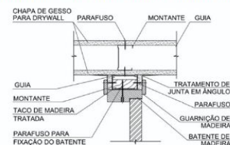
Figura 20 – Detalhe genérico esquemático – fonte: ABNT NBR 15758-1/2009
