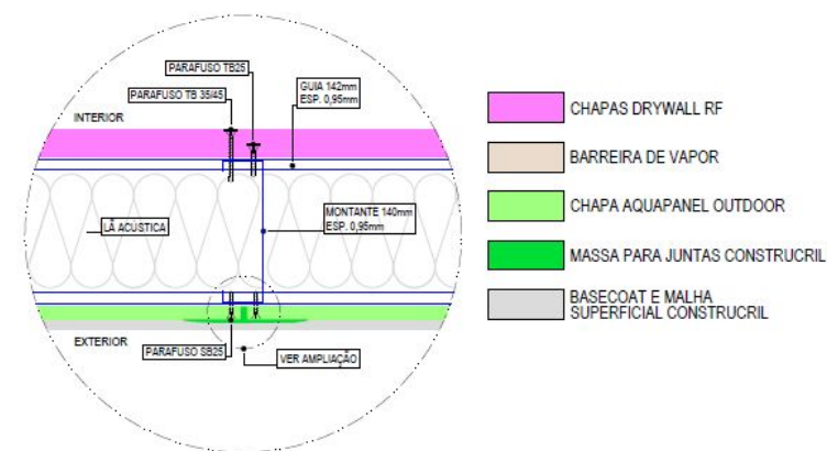
DETALHE A - Parede típica - Planta Esc. 1:5
