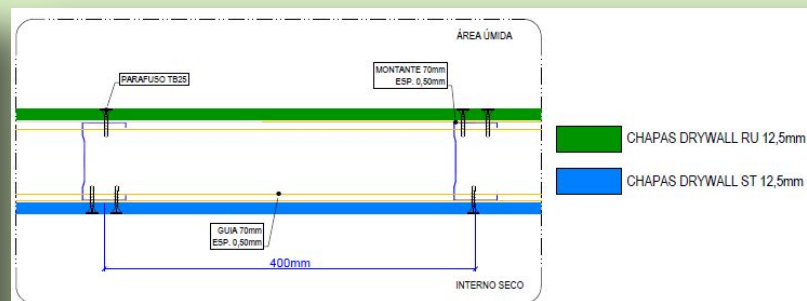
PAR TIPO 2 - Esp. 9,5cm - Planta
