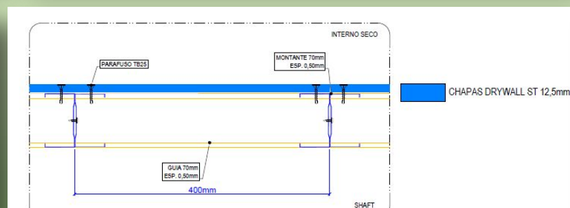
PAR TIPO 5 - Esp. 8,25cm - Planta
