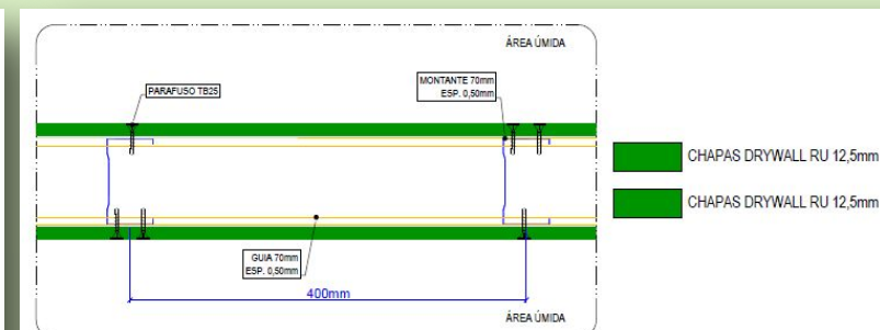
PAR TIPO 3 - Esp. 9,5cm - Planta
