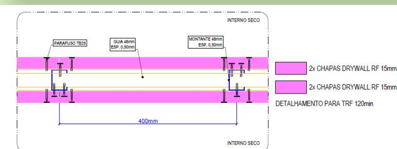
PAR TIPO 4 - Esp. 10,8cm - Planta
