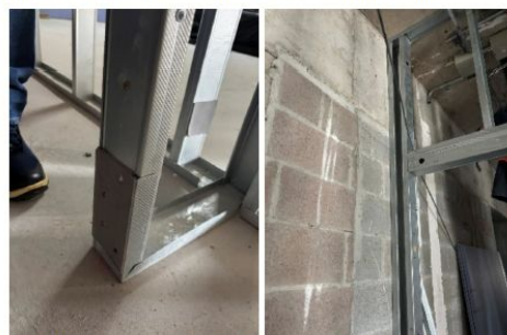
Figura 18 e 19 – Fixação do montante na guia inferior e reforço com montante duplo e madeira tratada
