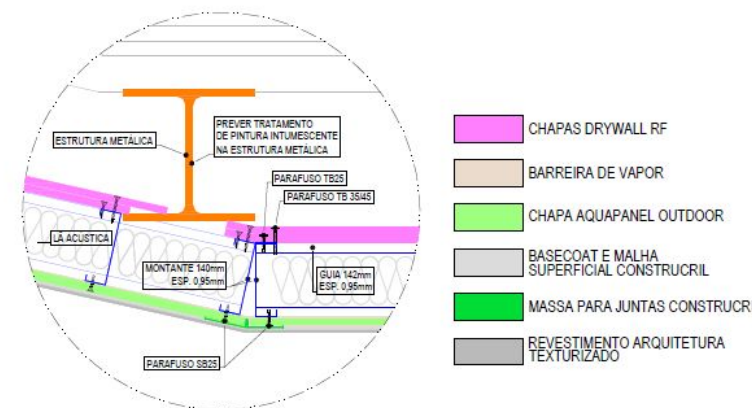
DETALHE H - Canto em angulação - Planta
